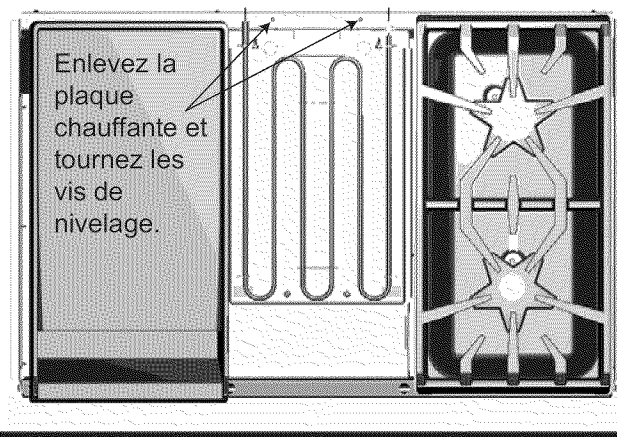
Figure 25 : Vis de nivelage de la plaque chauffante
